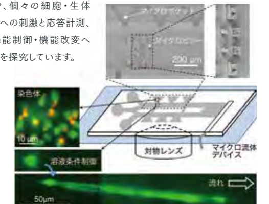
個々の細胞からの染色体取り出しおよび染色体1分子解析が可能なマイクロ流体デバイスの開発
