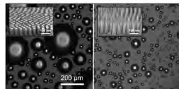
ナノスケール構造を持つメタ材料による防曇界面
