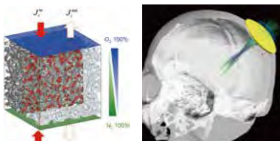
▲固体高分子形燃料電池内部の流れの解析 ▲スーパーコンピュータによる生体力学シミュレーション
